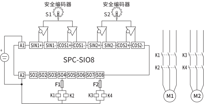
输入元件：S1（编码器）；S2（编码器） 控制逻辑：S1 & S2（速度监控） 安全等级：Cat.4 性能等级：PLe 安全完整性等级：SIL3
